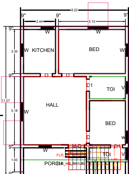
G.F PLAN
