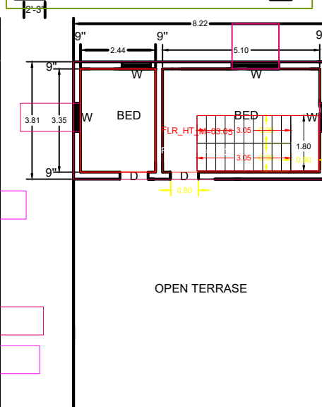
F.F PLAN
