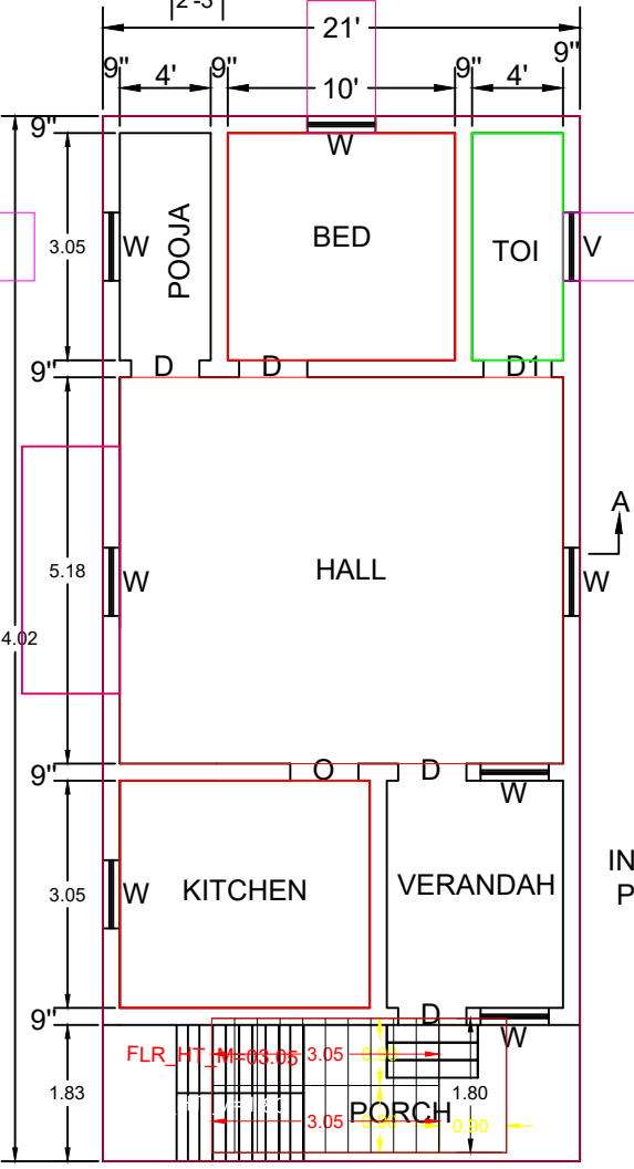
F.F PLAN
