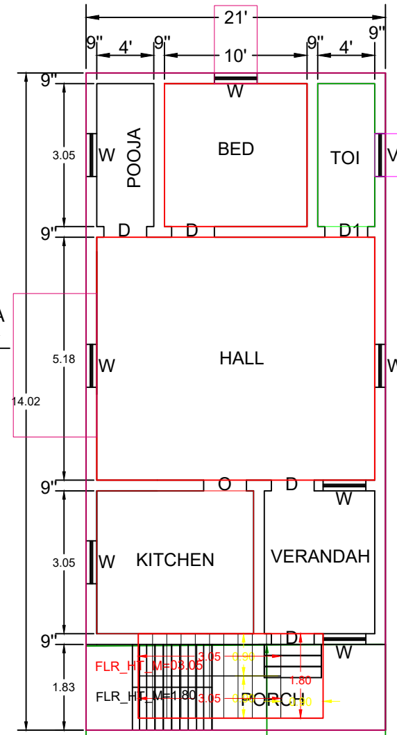
G.F PLAN
