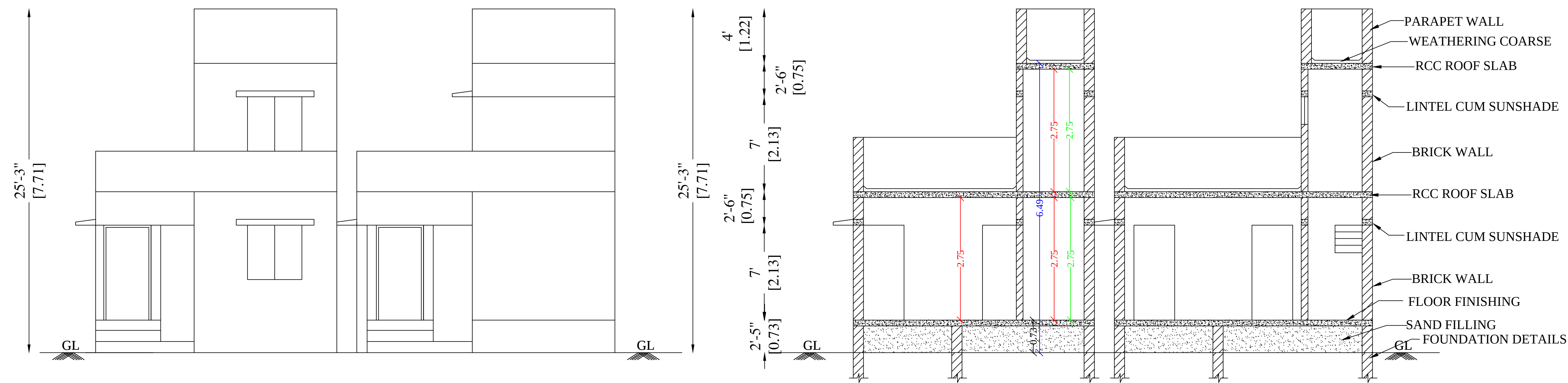
ELEVATION
