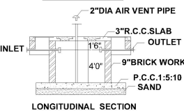
LONGITUDINAL SECTION
