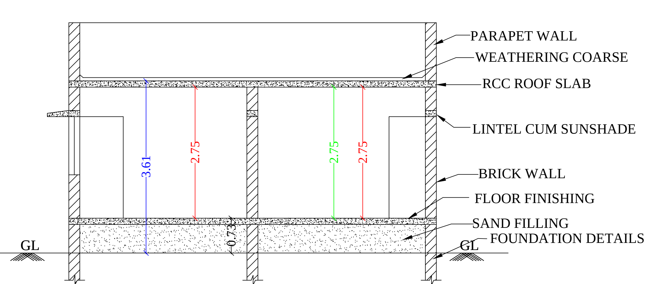
SECTION A-A
