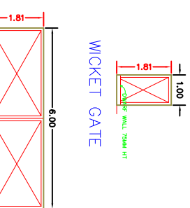
NTS
