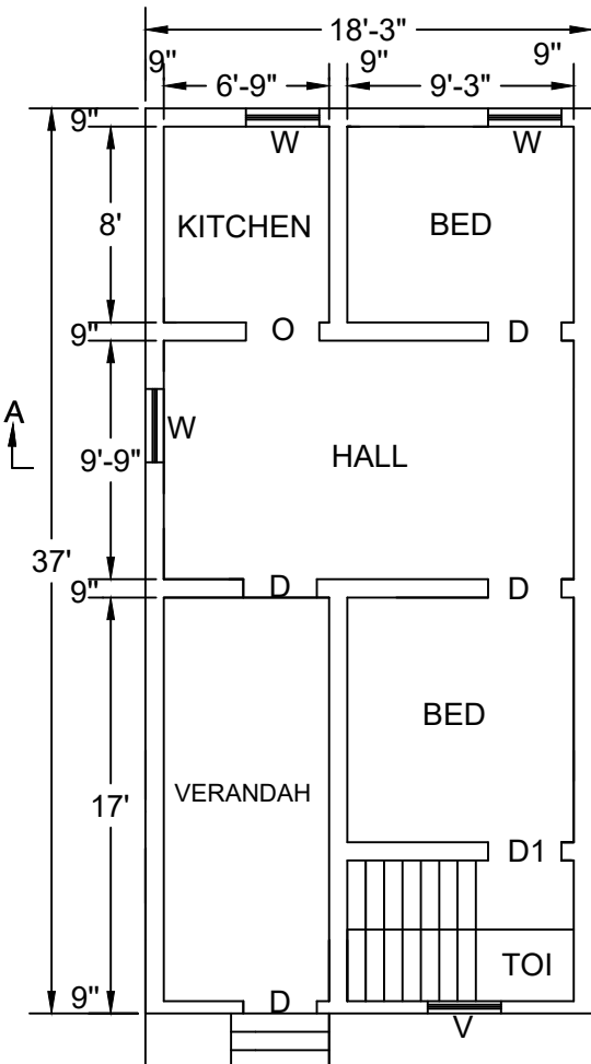
G.F.RESI PLAN
