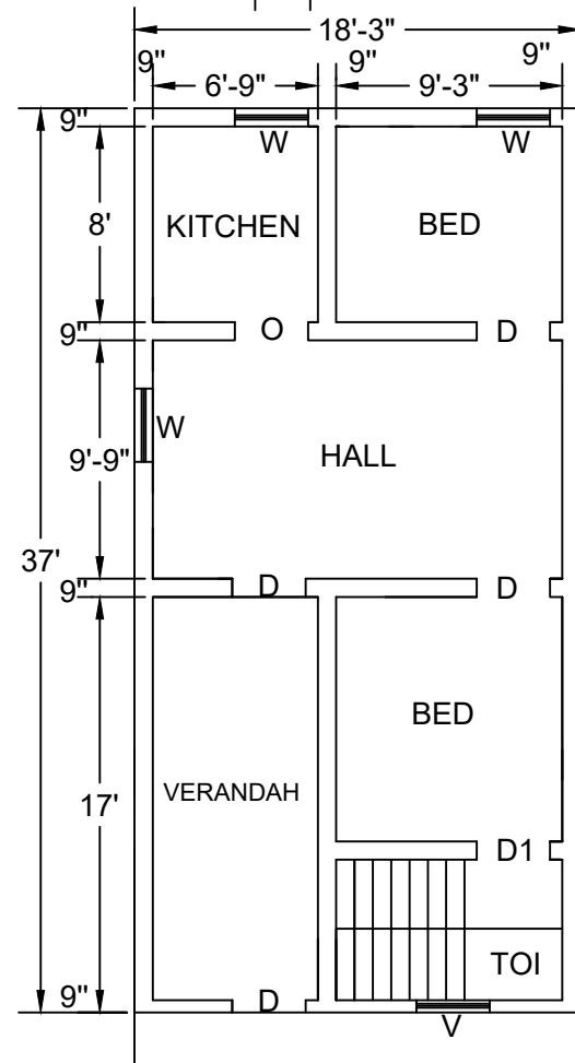
F.F.RESI PLAN
