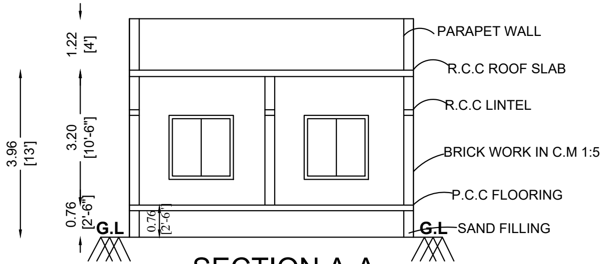
SECTION A-A
