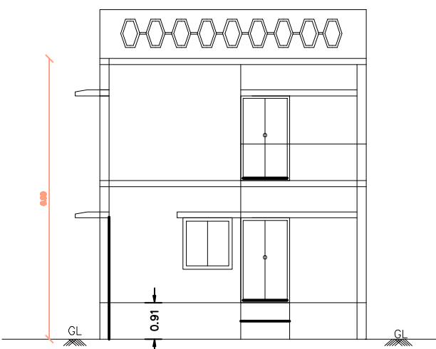
ELEVATION
