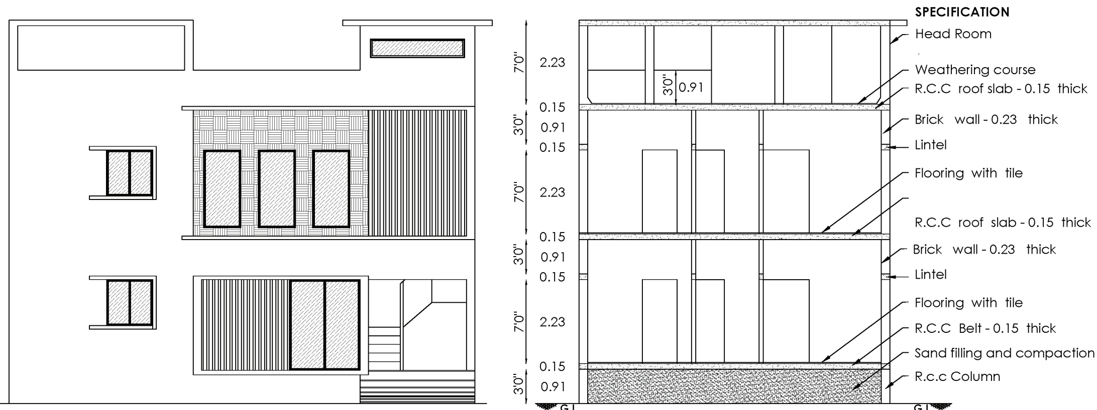
ELEVATION
