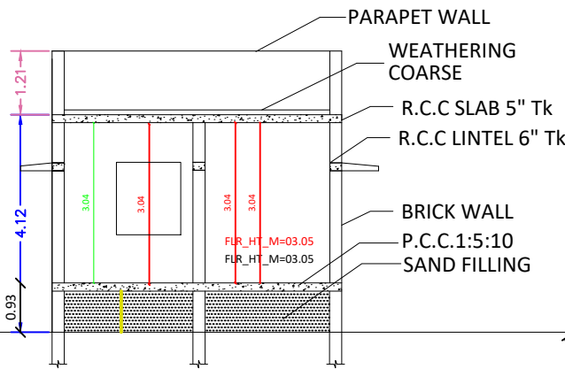
SECTION -AB
