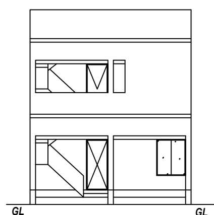
ELEVATION
