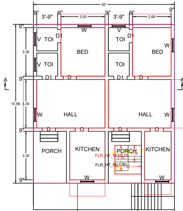
G.F PLAN
