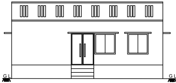
ELEVATION
