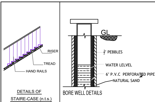
DETAILS OF STAIRCASE (n.t.s.)
