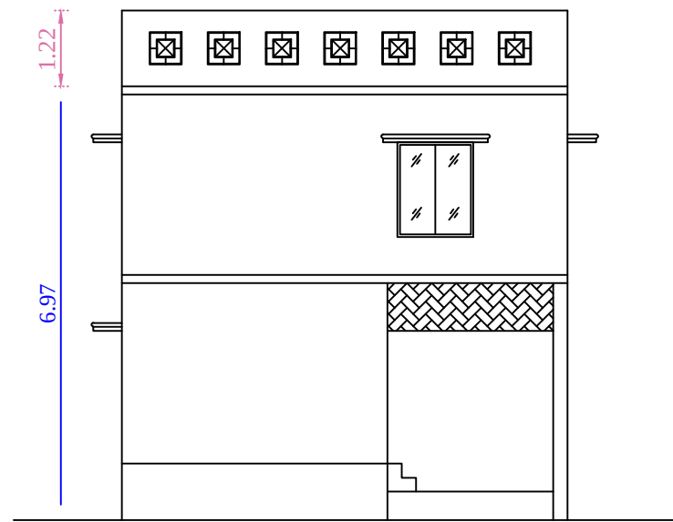
ELEVATION
