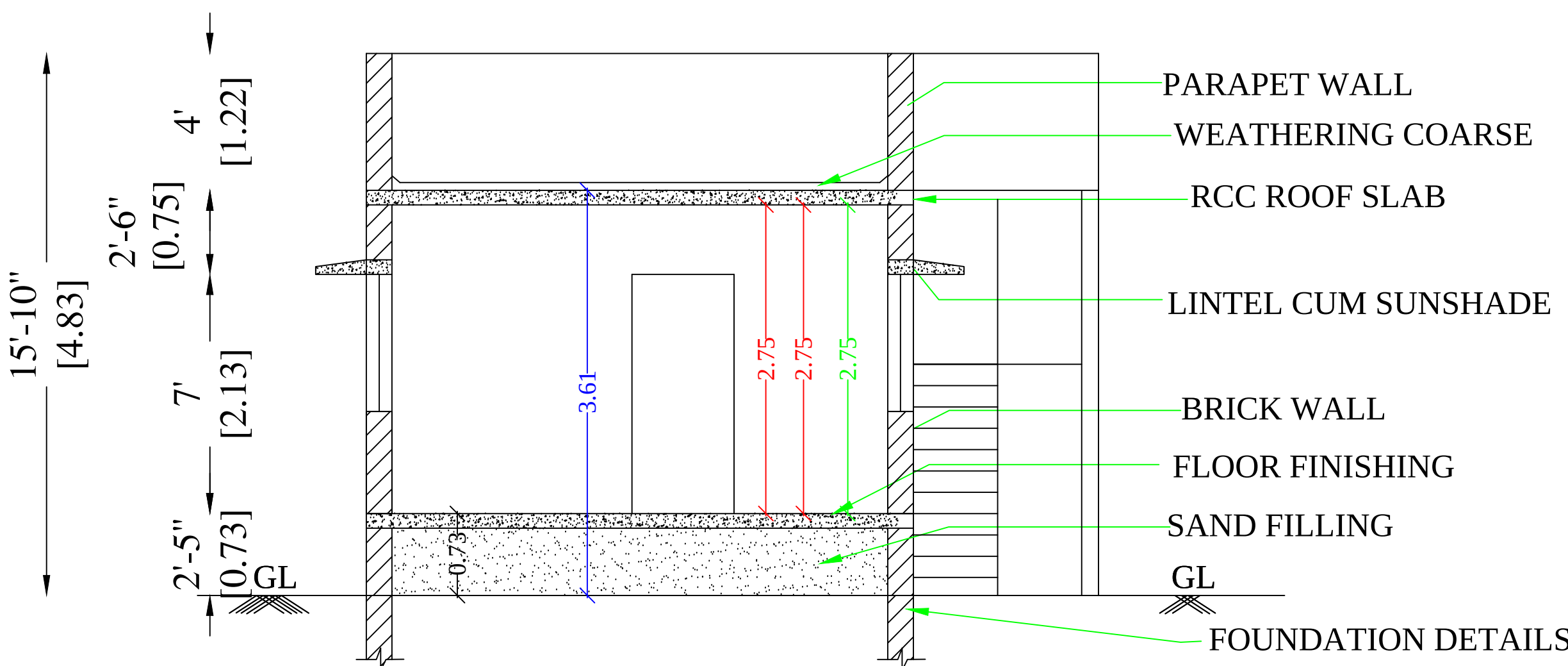
SECTION A-A
