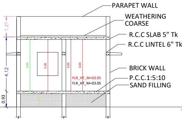
SECTION -AB
