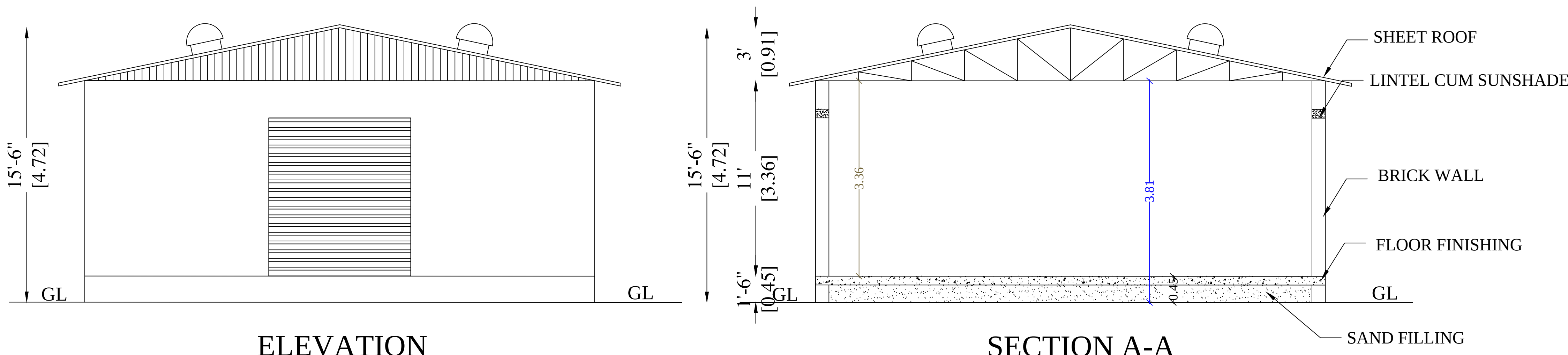
ELEVATION
