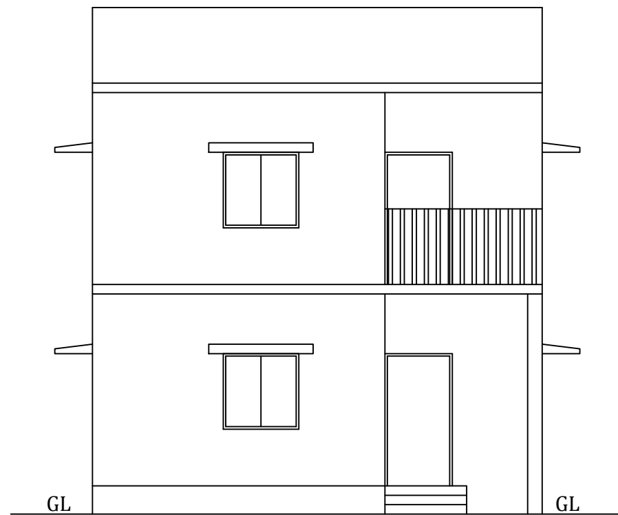
ELEVATION
