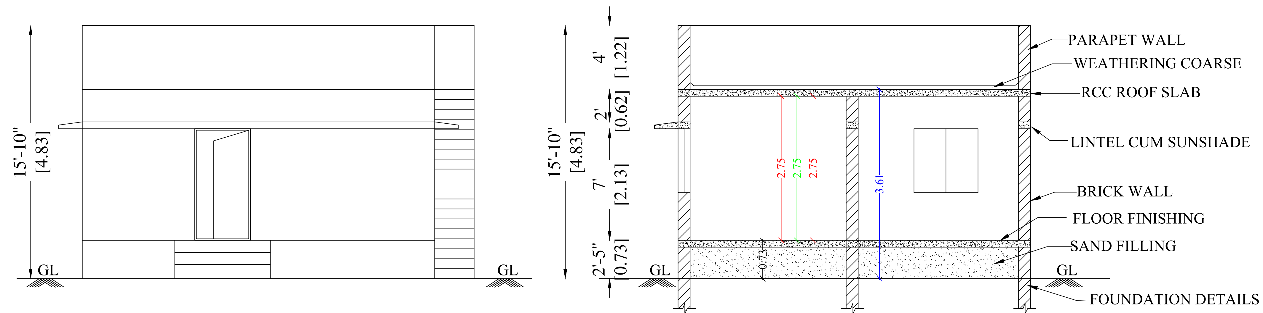
ELEVATION
