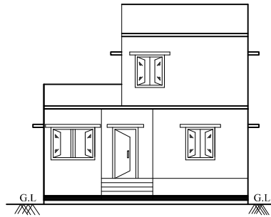
ELEVATION
