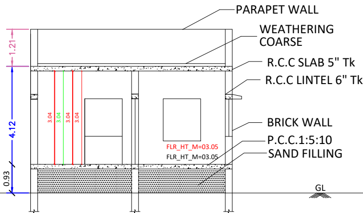
SECTION -AB
