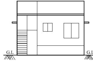
ELEVATION
