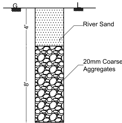
RAIN WATER STORAGE (N.T.S)
