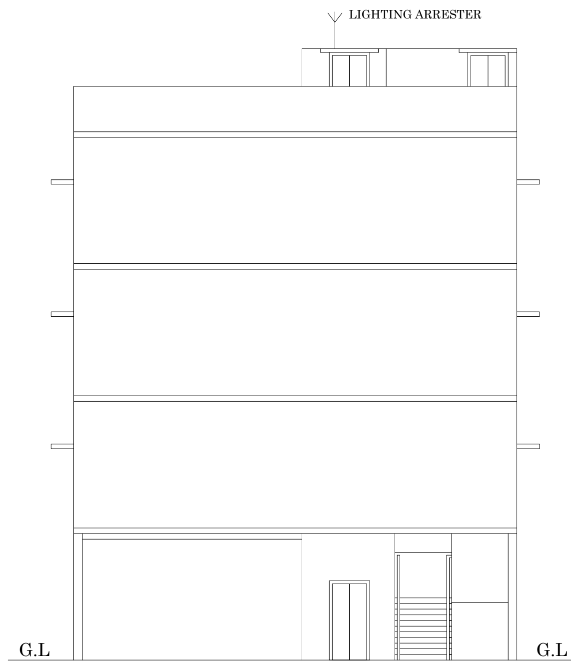
ELEVATION
