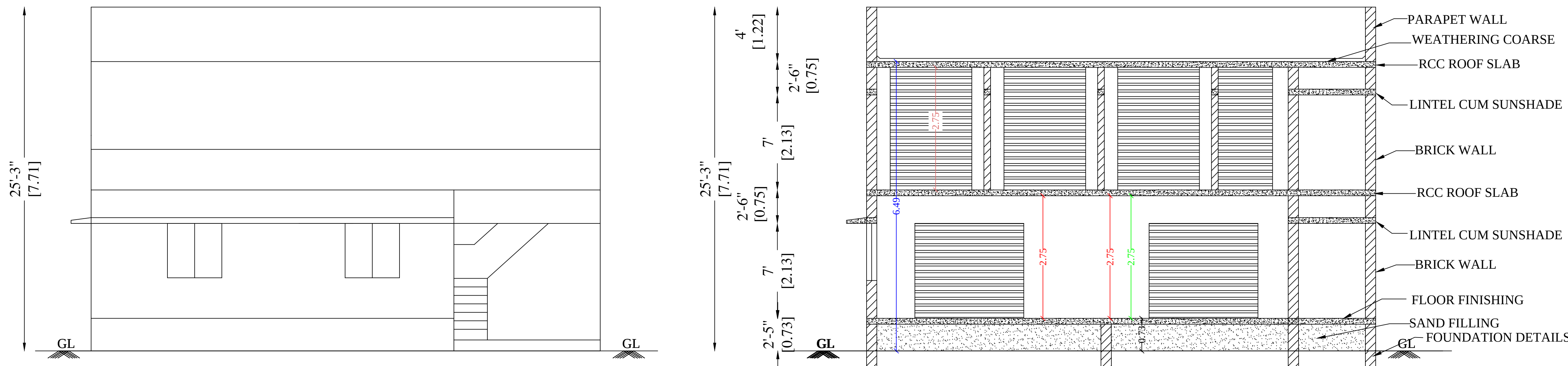
ELEVATION
