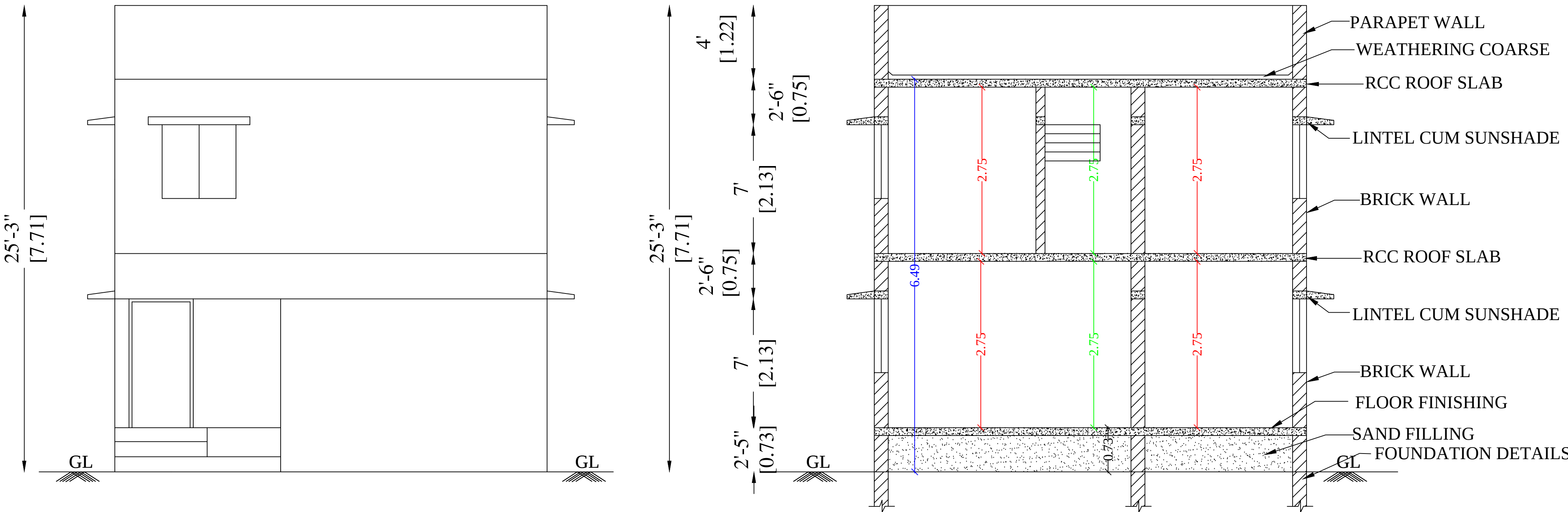
ELEVATION
