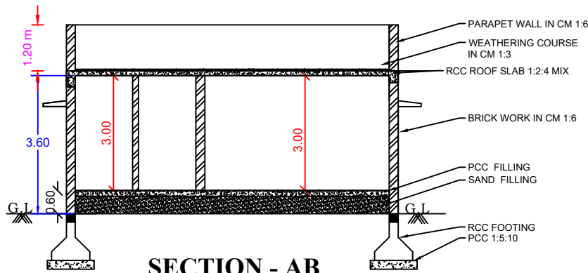
SECTION - AB
