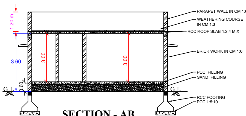
SECTION - AB
