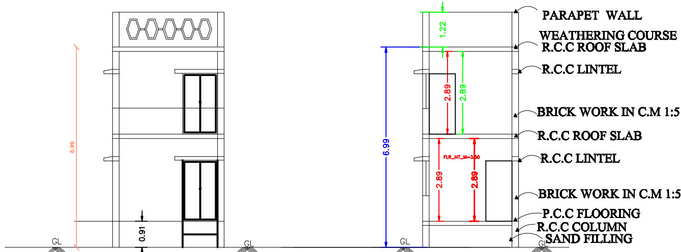
ELEVATION
