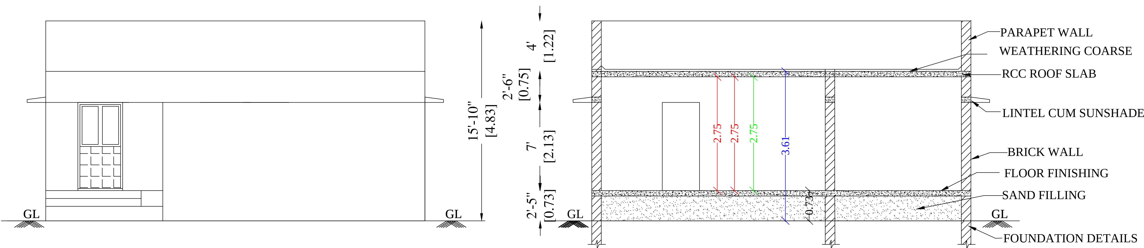
ELEVATION
