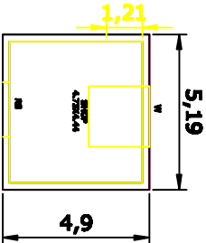
ELEVATION
