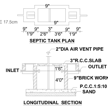
LONGITUDINAL SECTION
