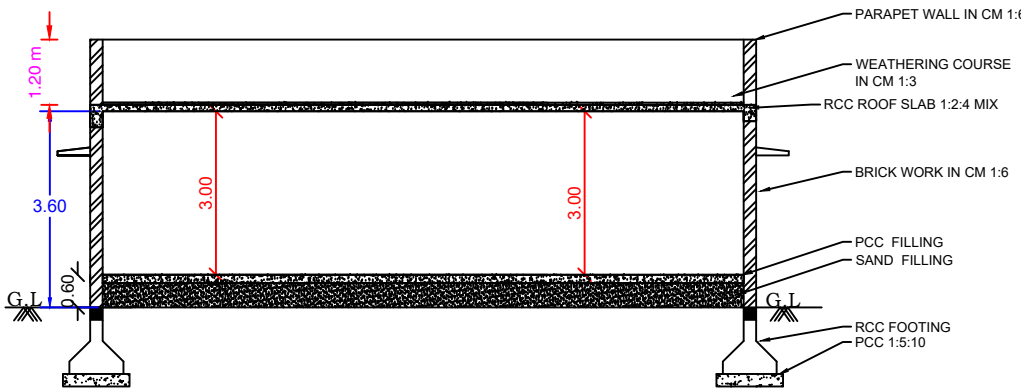
SECTION - AB
