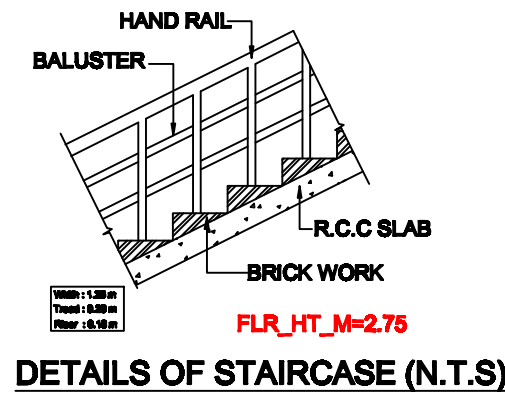
DETAILS OF STAIRCASE (N.T.S)
