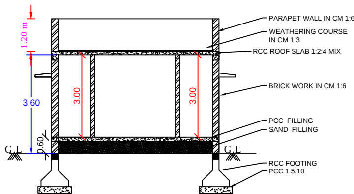
SECTION - AB
