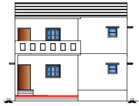
ELEVATION
