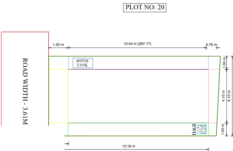
PLOT NO: 20
