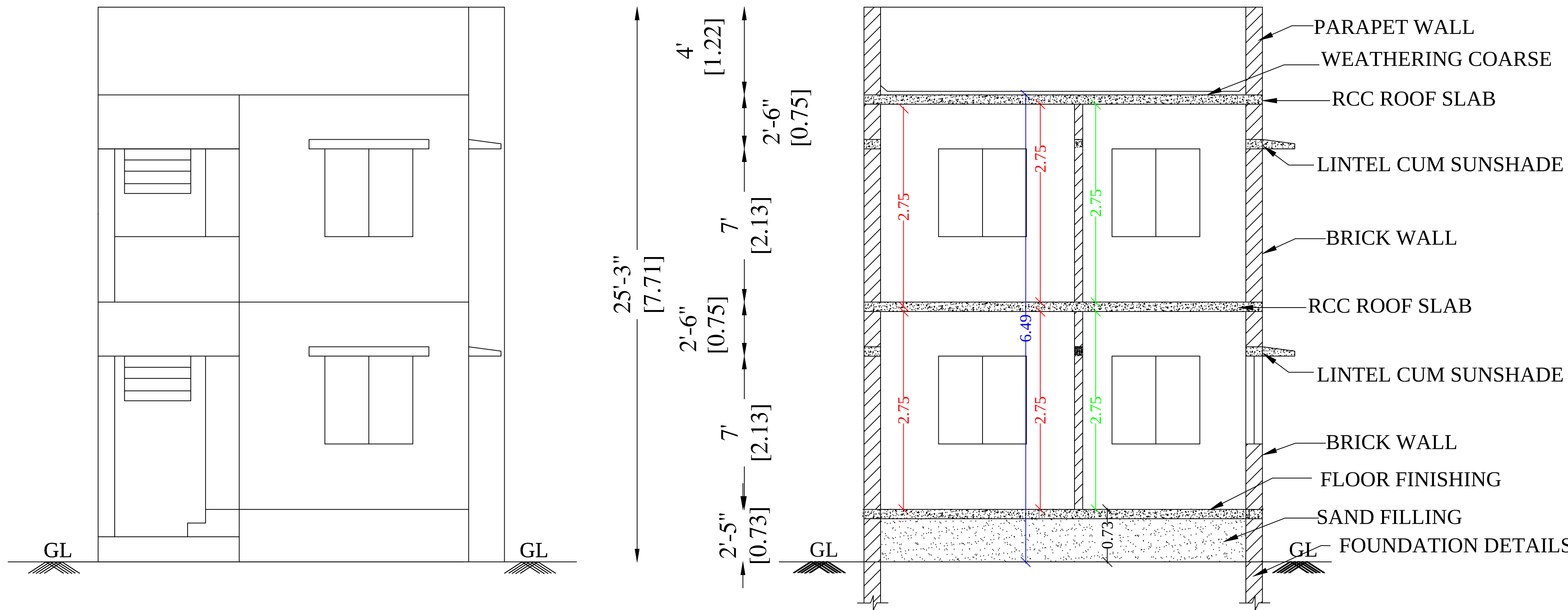
ELEVATION
