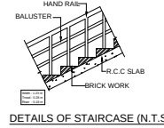
DETAILS OF STAIRCASE (N.T.S.)
