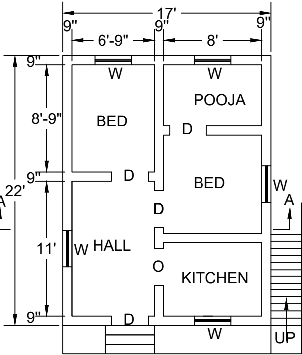
G.F PLAN
