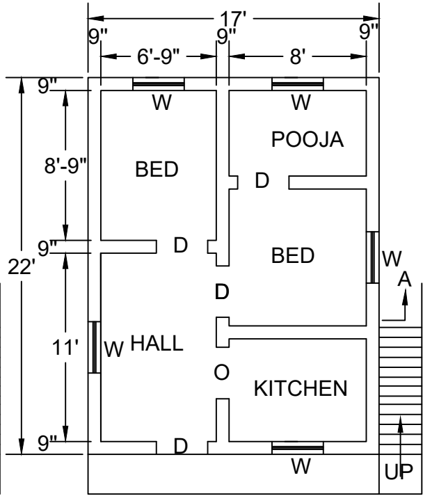
F.F PLAN
