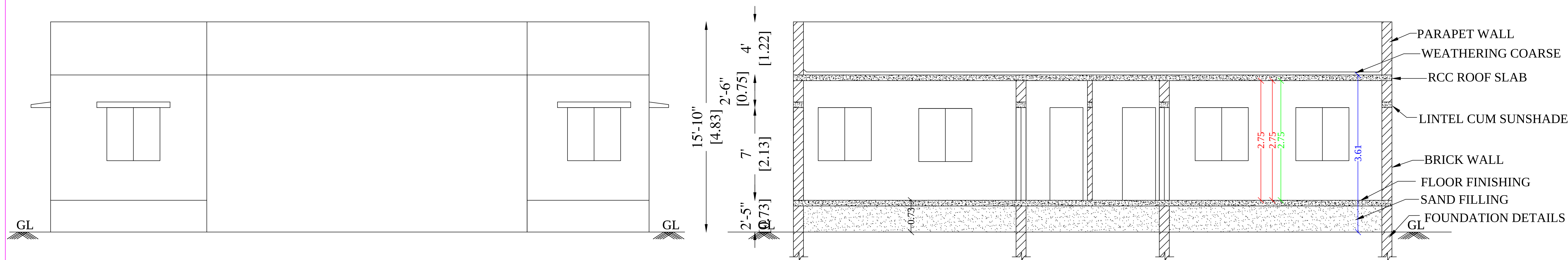
ELEVATION
