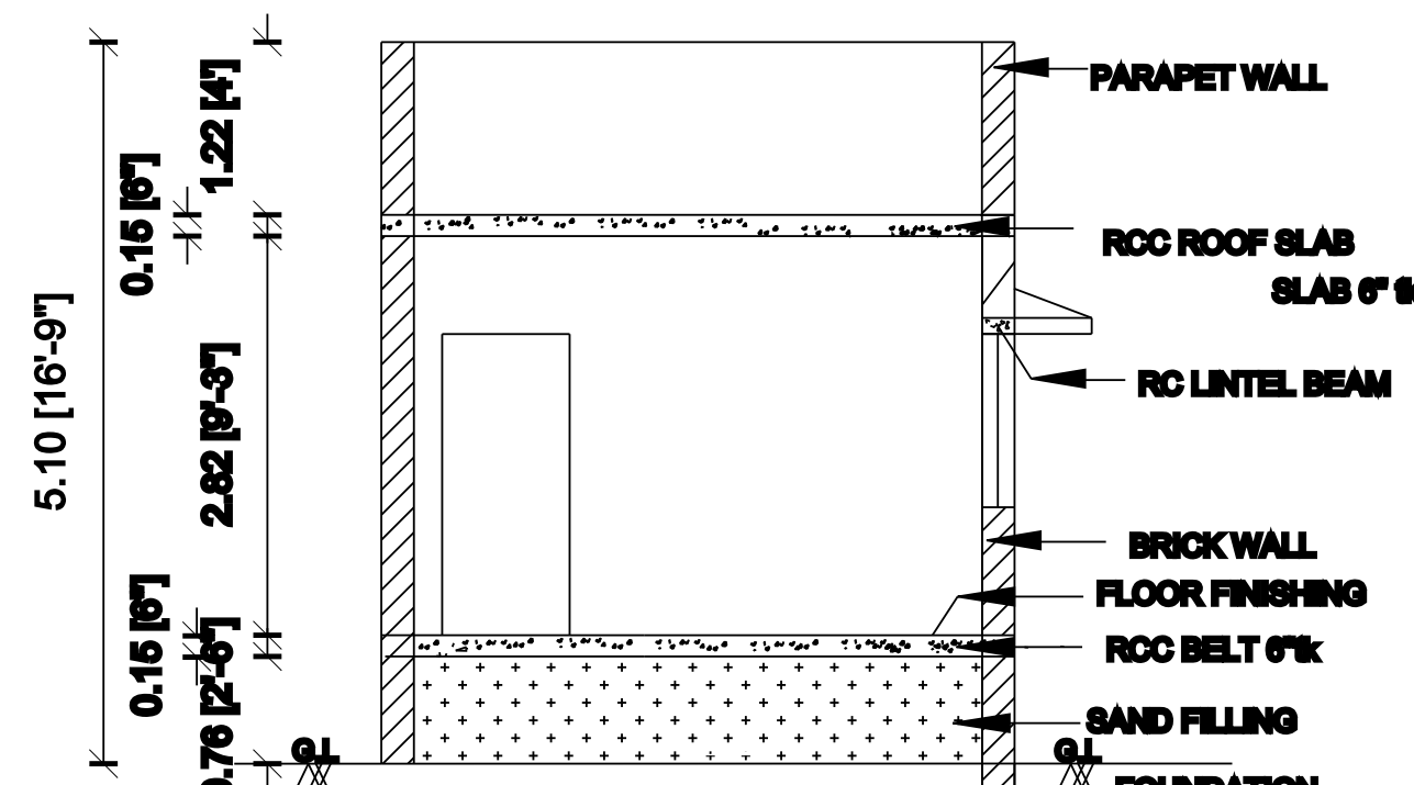
SECTION A-A
