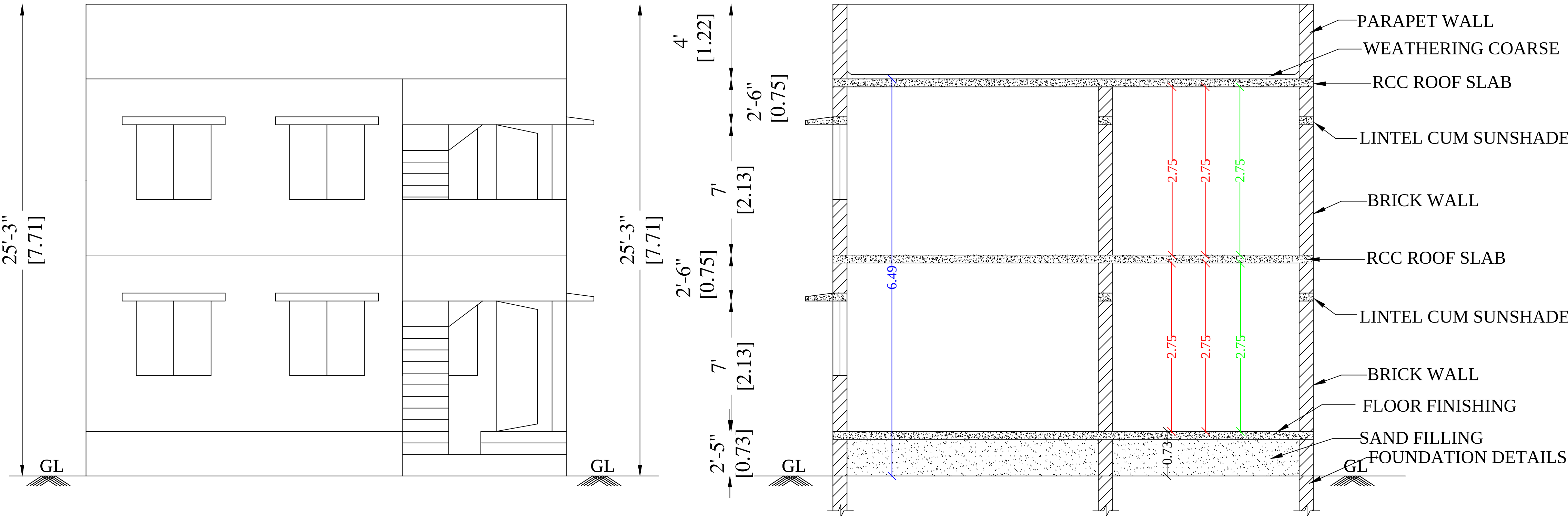
ELEVATION
