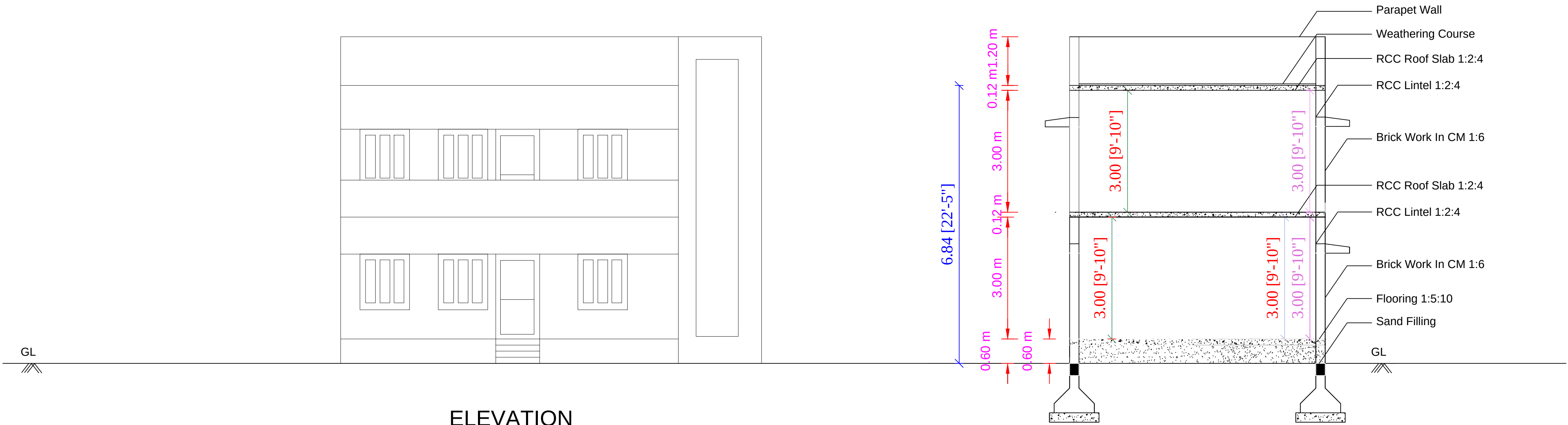
ELEVATION
