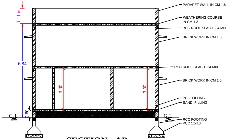
SECTION - AB
