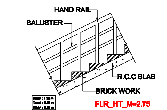
DETAILS OF STAIRCASE (N.T.S)
