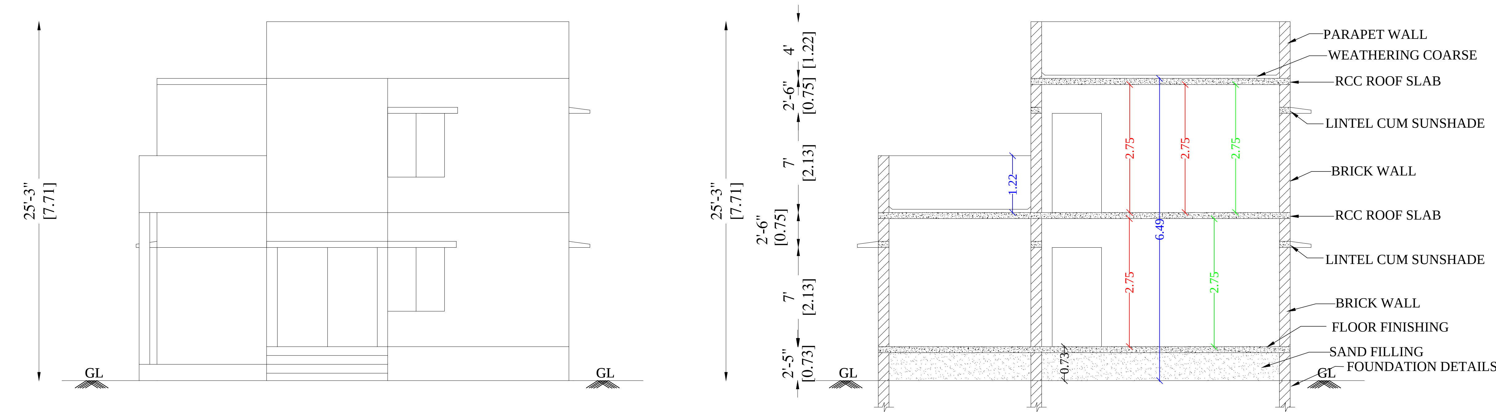
ELEVATION
