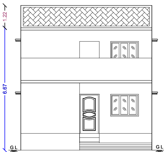
ELEVATION
